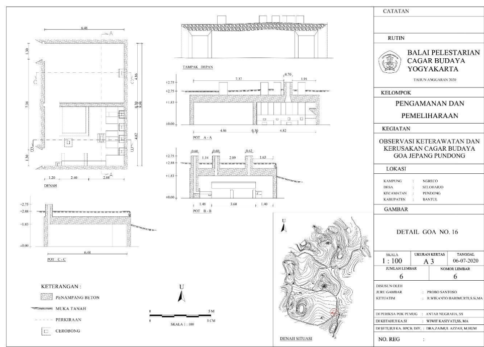
Gambar Denah potongan Gua Jepang Nomor 16 (Sumber: Balai Pelestarian Cagar Budaya Daerah Istimewa Yogyakarta, 2021)
