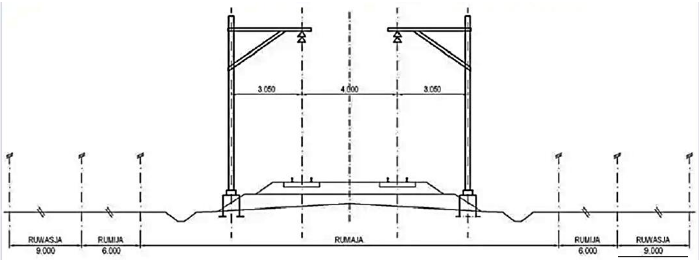
Penampang melintang Ruang Jalur Kereta api Permukaan Tanah Jalur Ganda
