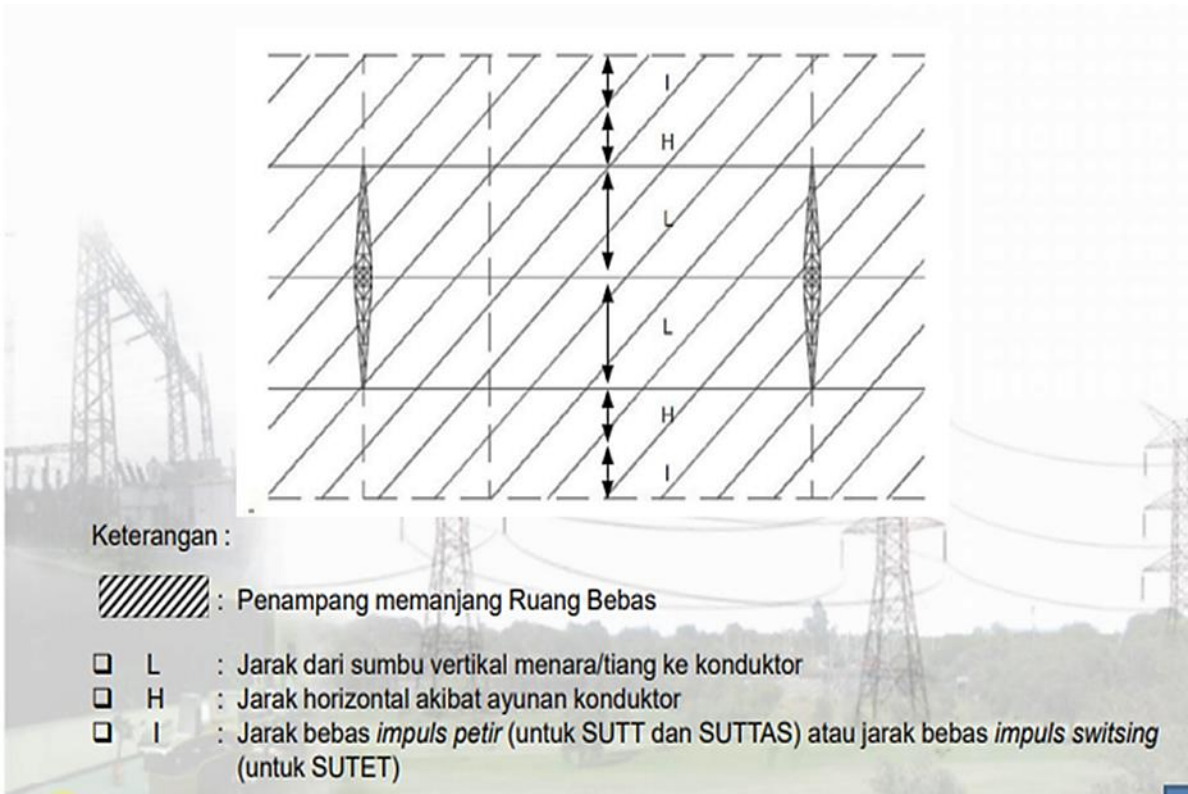
Gambar Penampang memanjang Ruang Bebas Jarak Minimum Horisontal
