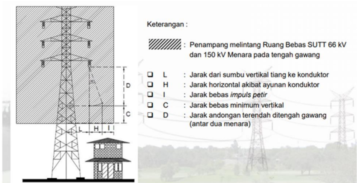
Gambar Penampang Ruang Bebas pada SUTT 66kV dan 150kV Menara
