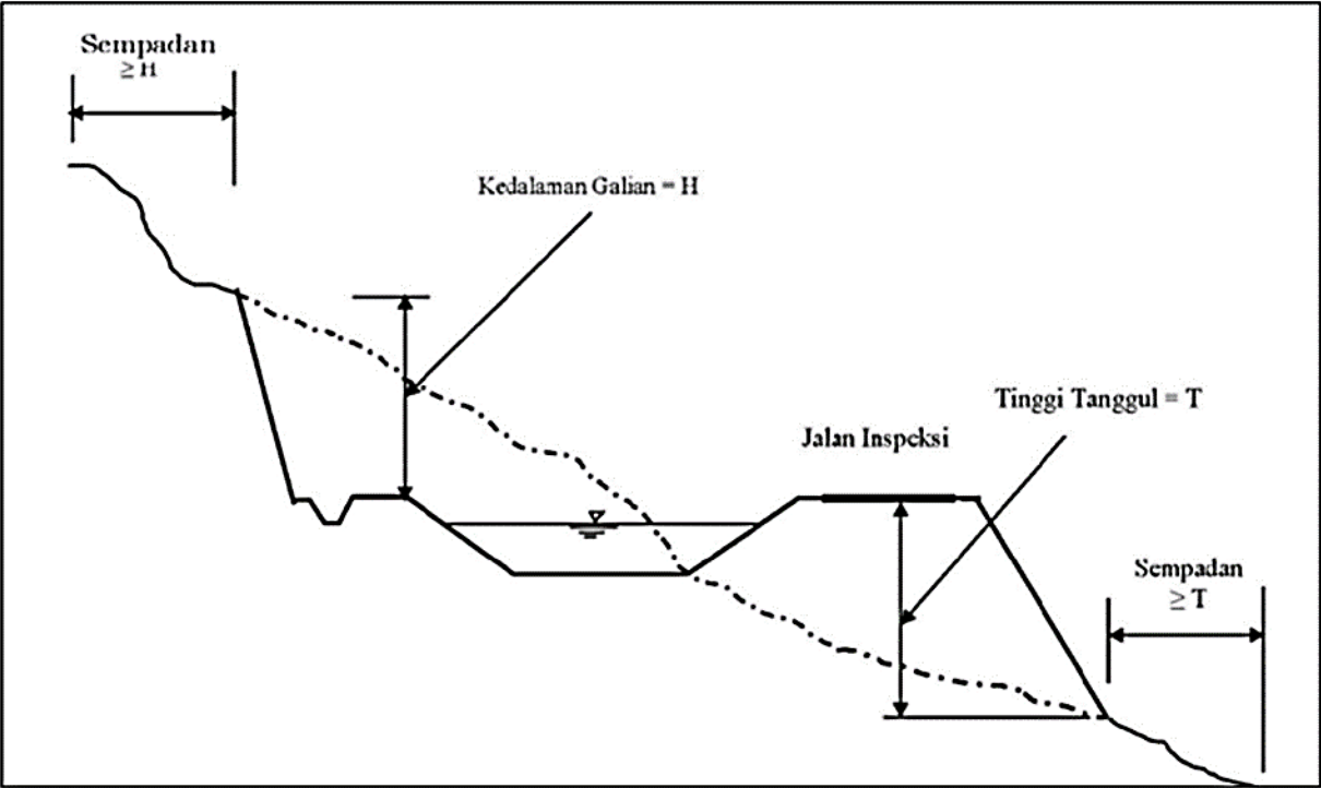
Penampang Garis Sempadan Jaringan Irigasi pada lereng atas dan bawah jaringan irigasi
