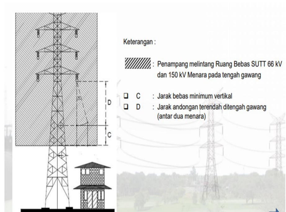
Gambar Penampang memanjang Ruang Bebas Jarak Minimum Vertikal
