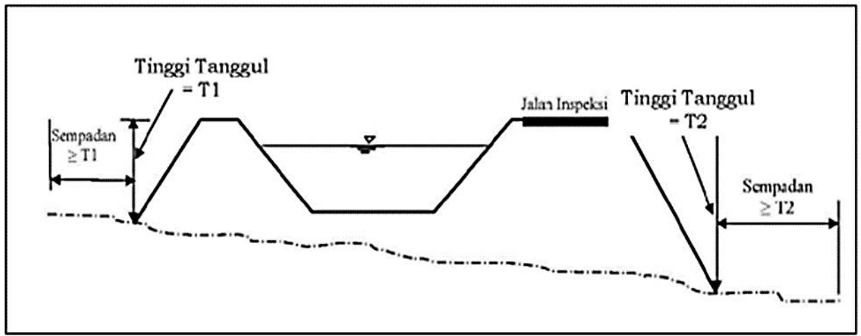
Penampang Garis Sempadan Jaringan Irigasi Bertanggul
