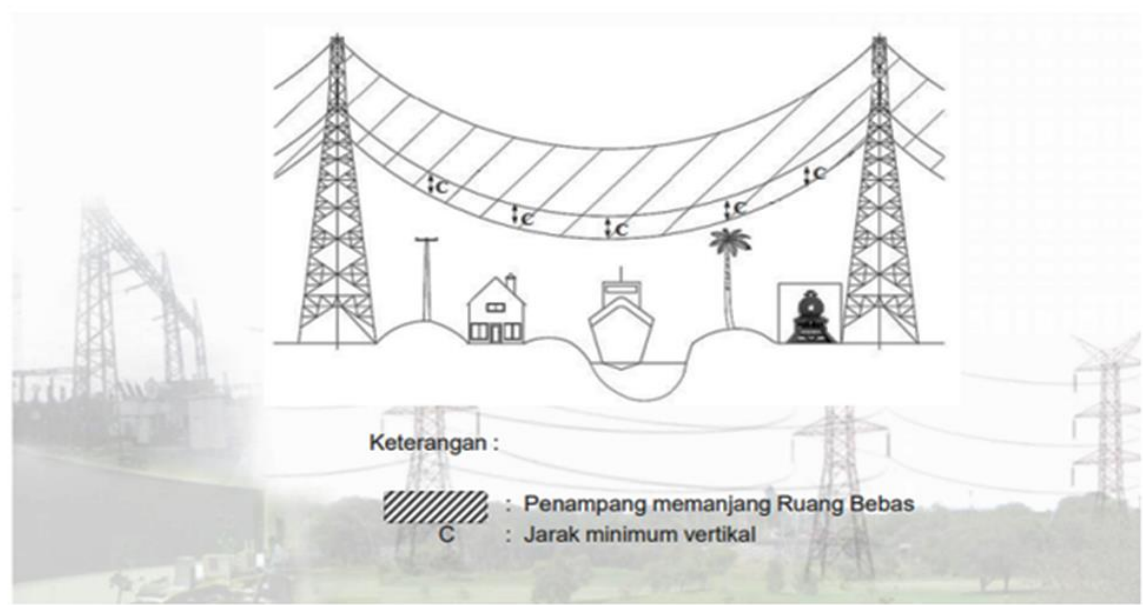
Gambar Penampang memanjang Ruang Bebas Jarak Minimum Vertikal
