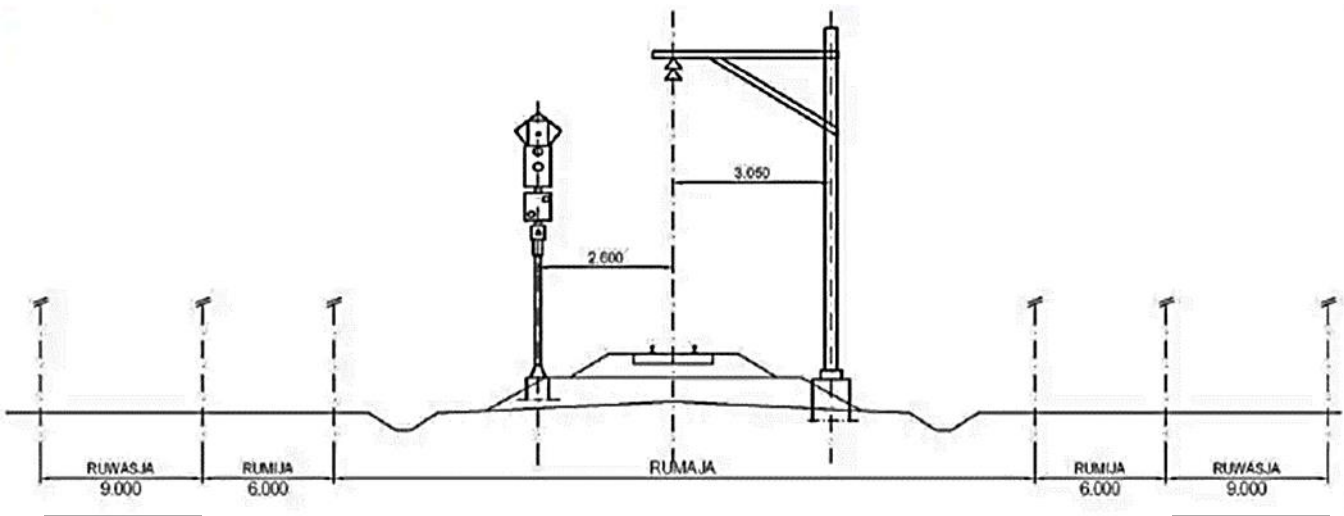
Penampang melintang Ruang Jalur Kereta Api Permukaan Tanah Jalur Tunggal
