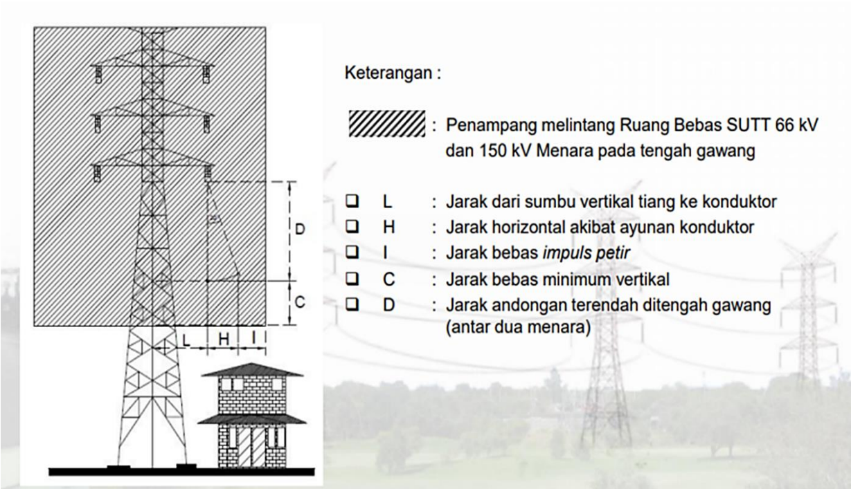
Gambar Penampang Ruang Bebas SUTT 66 kV dan 150kV Menara Tabel Jarak Bebas Minimum Horizontal dari Sumbu Vertikal Menara/Tiang pada SUTT, SUTET dan SUTTAS
