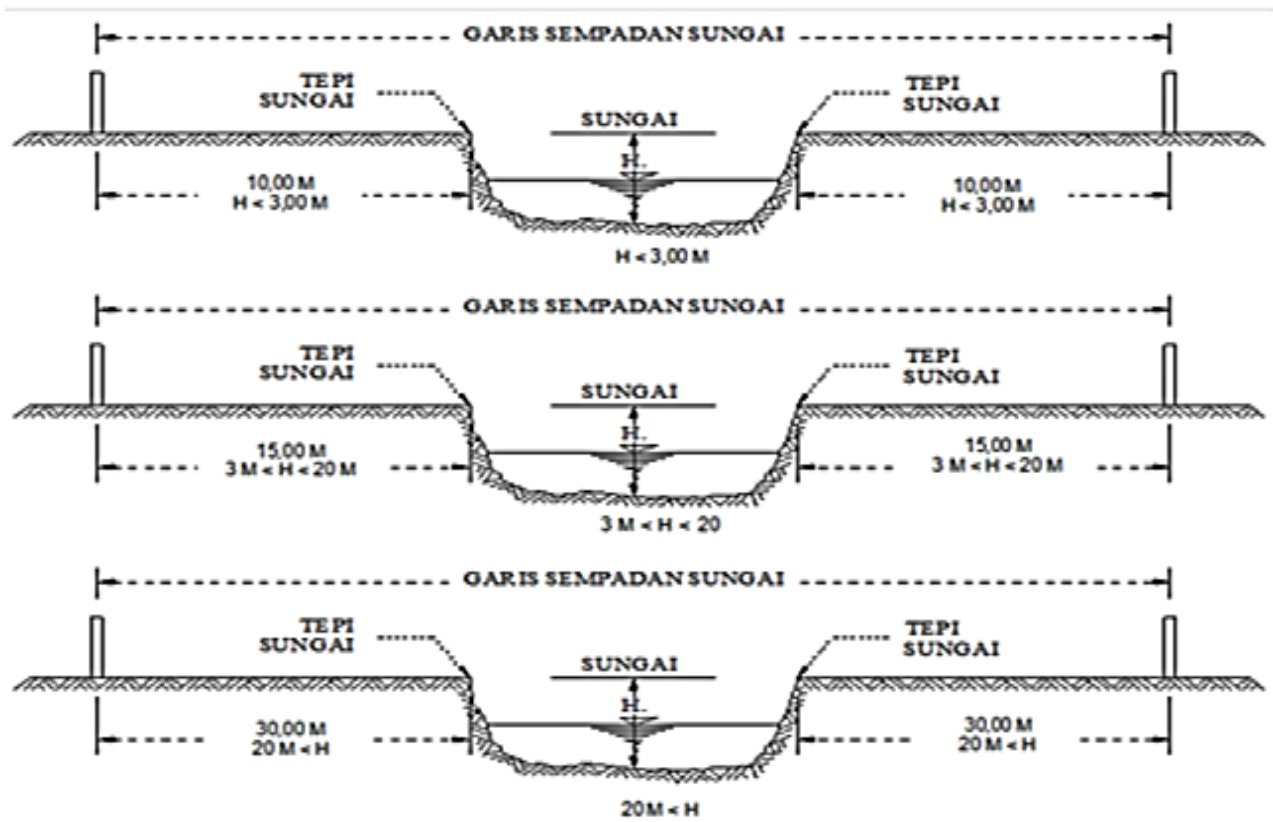
Penampang Garis Sempadan Sungai Tidak Bertanggul di Dalam Kawasan Perkotaan
