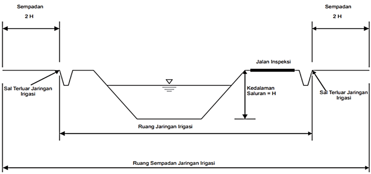
Penampang Garis Sempadan Jaringan Irigasi Tidak Bertanggul
