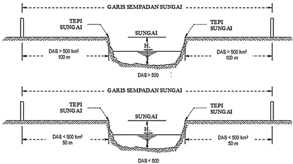
Penampang Garis Sempadan Sungai Tidak Bertanggul di Luar Kawasan Perkotaan
