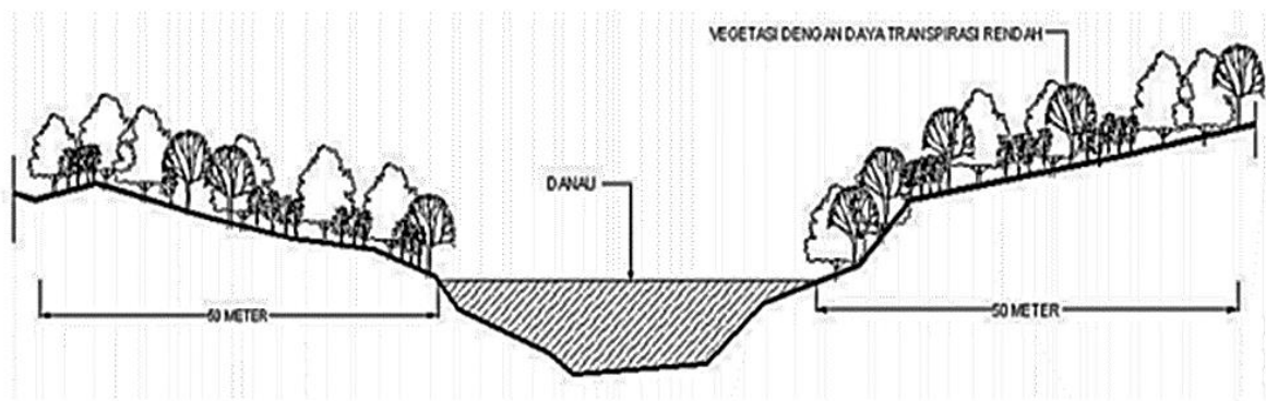
Penampang Sempadan Embung dengan jarak 50 meter
